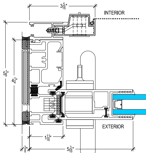
LOCK JAMB
