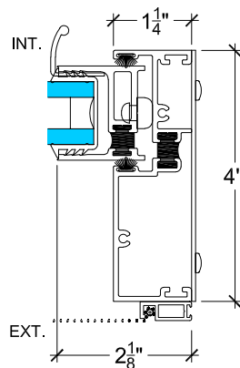
LATCH JAMB
