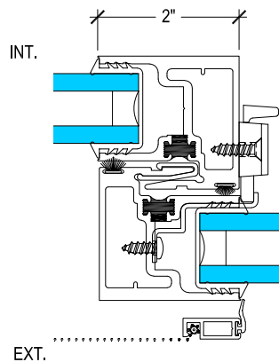
INTERLOCKER
