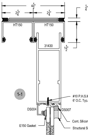
OPTIONAL 1 1/16" GLASS
