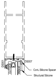
OPTIONAL 1 1/16" GLASS
