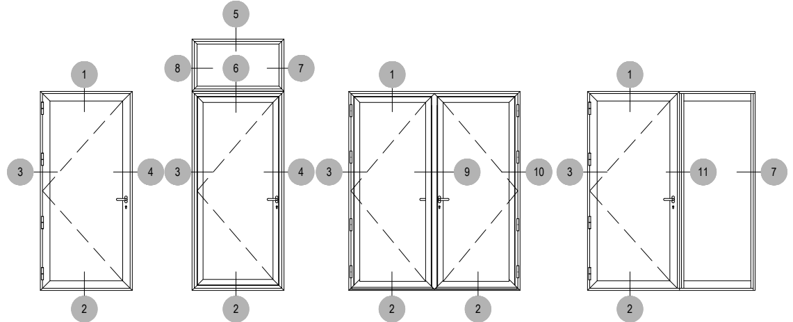
EXTERIOR ELEVATION N.T.S.
