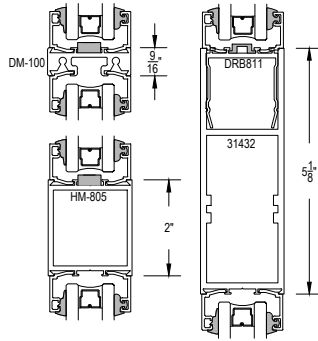
OPTIONAL HORIZONTAL MUNTIN
