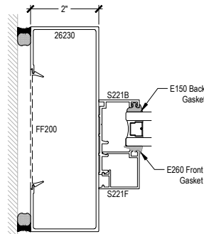
JAMB @ TRANSOM
