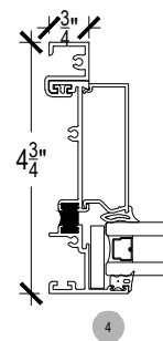
LEFT FIXED TRANSOM JAMB
