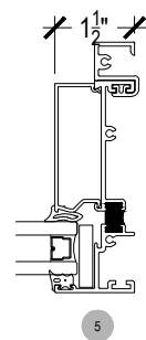
RIGHT FIXED TRANSOM JAMB
