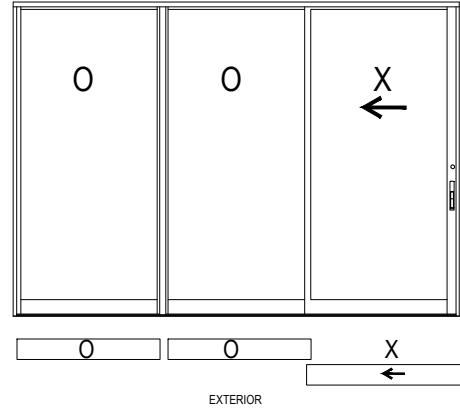
OOX CONFIGURATION
