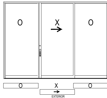
OLXO CONFIGURATION
