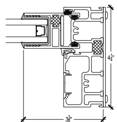
7 FIXED JAMB
