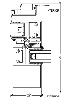
4 INTERLOCKERS
