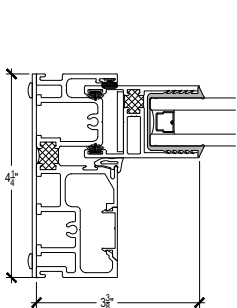
3 FIXED JAMB
