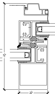
6 INTERLOCKERS
