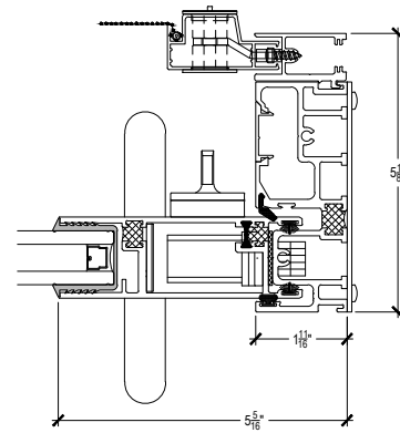
5 LATCH JAMB
