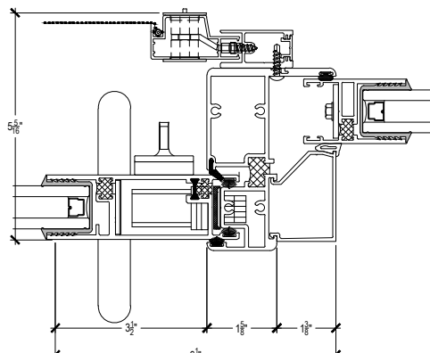
5 B-JAMB
