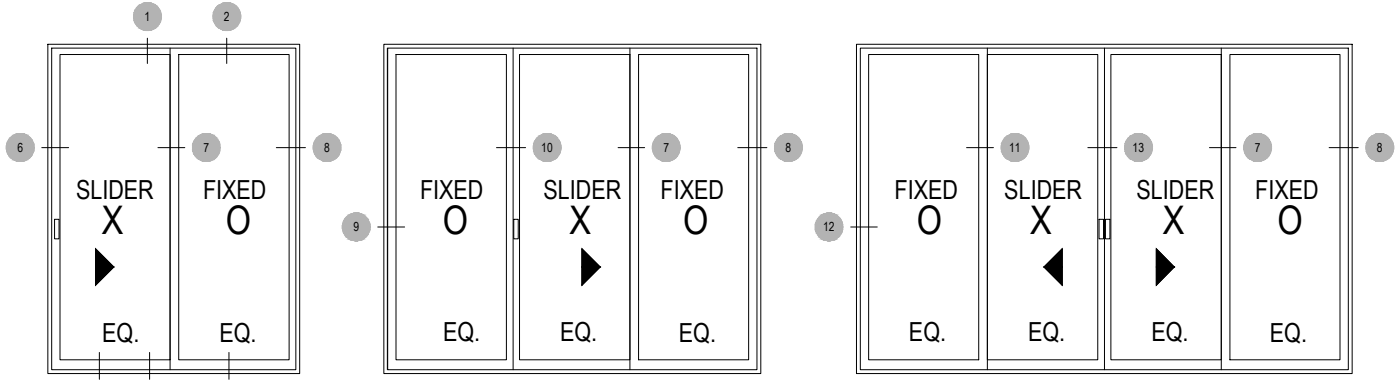
EXTERIOR ELEVATION N.T.S.
