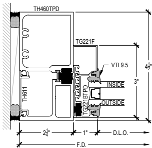
OPTIONAL THERMAL DOOR JAMB @ TRANSOM
