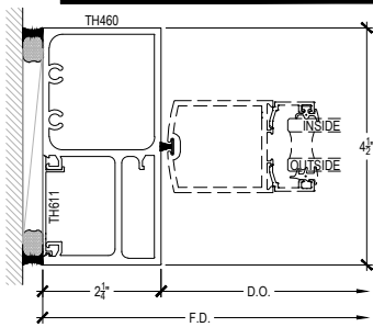
DOOR JAMB
