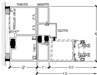
OPTIONAL THERMAL SUBFRAME DOOR JAMB
