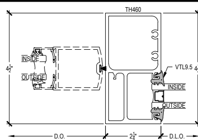
DOOR JAMB @ SIDELITE
