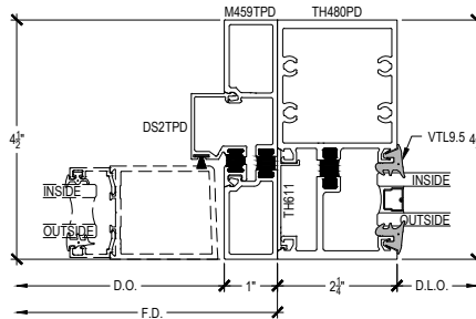
OPTIONAL THERMAL SUBFRAME DOOR JAMB @ SIDELITE
