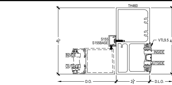
DOOR JAMB @ SIDELITE
