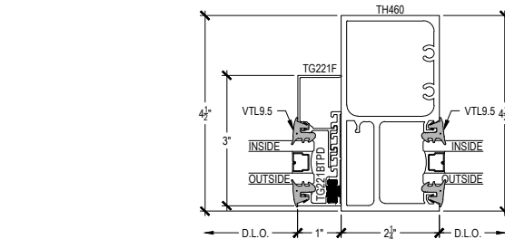
DOOR JAMB @ SIDELITE TRANSOM
