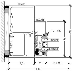
DOOR JAMB @ TRANSOM
