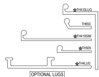
OPTIONAL LUGS
