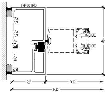
OPTIONAL THERMAL DOOR JAMB
