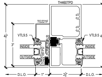
OPTIONAL THERMAL DOOR JAMB @ SIDELITE TRANSOM
