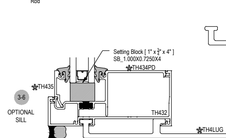
OPTIONAL LUGS
