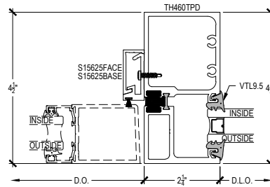
OPTIONAL THERMAL DOOR JAMB @ SIDELITE
