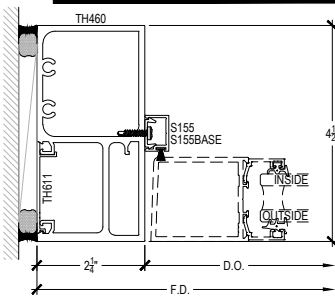
DOOR JAMB
