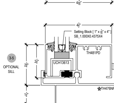
OPTIONAL SILL
