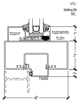
9-1 HORIZONTAL @ OFFSET DOOR
