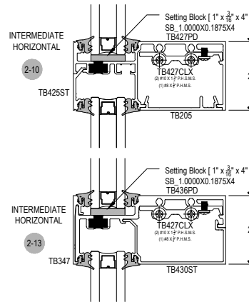
Top Load
