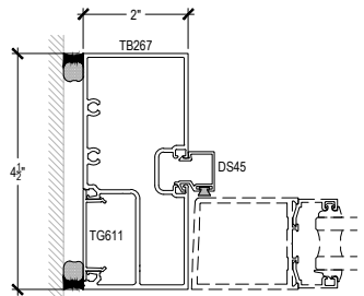
DOOR JAMB @ OFFSET DOOR WITHOUT TRANSOM
