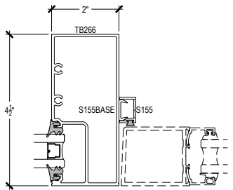
DOOR JAMB @ OFFSET DOOR
