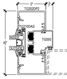
DOOR JAMB W/SIDELITE @ OFFSET DOOR
