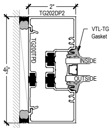
WALL JAMB
