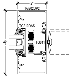
DOOR JAMB W/SIDELITE @ CENTER DOOR
