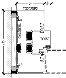
DOOR JAMB @ OFFSET DOOR
