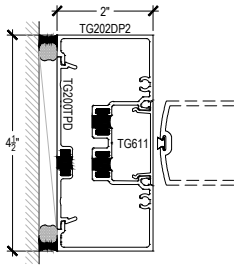
DOOR JAMB @ CENTER DOOR
