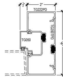
7-4 JAMB @ OFFSET DOOR
