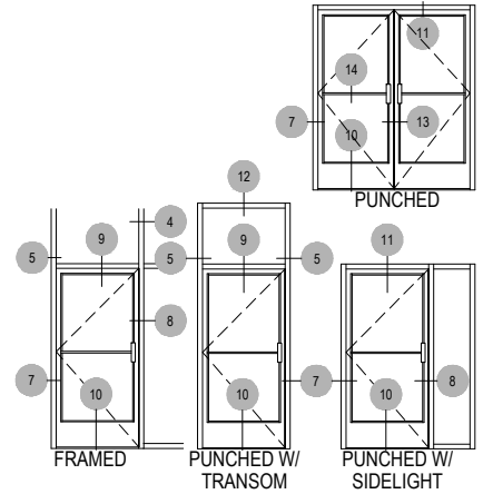
7-5 OPTIONAL JAMB @ CENTER DOOR
