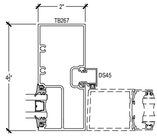
DOOR JAMB @ OFFSET DOOR WITHOUT TRANSOM
