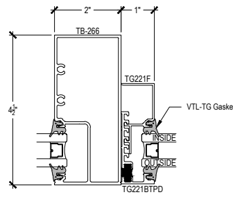
OPTIONAL JAMB @ TRANSOM
