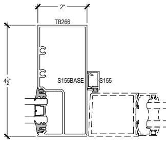
DOOR JAMB @ OFFSET DOOR
