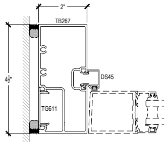
DOOR JAMB @ OFFSET DOOR WITHOUT TRANSOM
