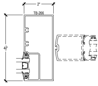
DOOR JAMB @ CENTER DOOR
