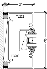
WALL JAMB
