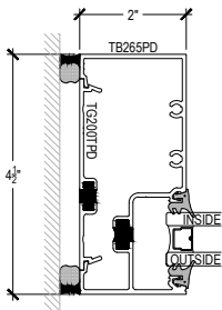
WALL JAMB
