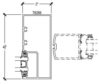
DOOR JAMB @ CENTER DOOR
