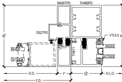
OPTIONAL THERMAL SUBFRAME DOOR JAMB @ SIDELITE 8-5
