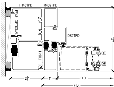
OPTIONAL THERMAL SUBFRAME DOOR JAMB 7-5
