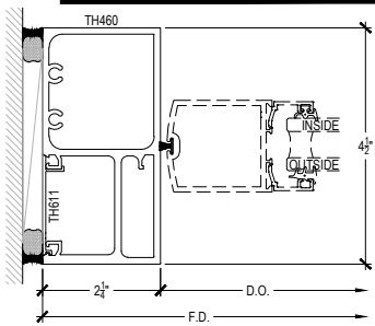
DOOR JAMB 7-3
