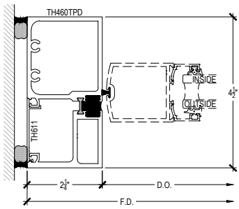
OPTIONAL THERMAL DOOR JAMB 7-4
