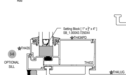
OPTIONAL LUGS
