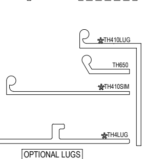
OPTIONAL LUGS
