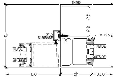
DOOR JAMB @ SIDELITE
