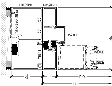
OPTIONAL THERMAL SUBFRAME DOOR JAMB
