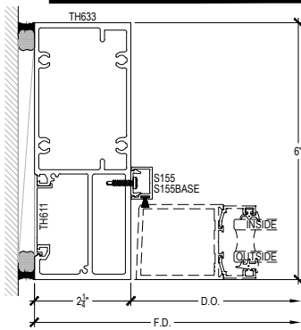
DOOR JAMB
