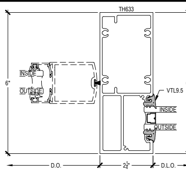
DOOR JAMB @ SIDELITE
