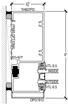
JAMB
