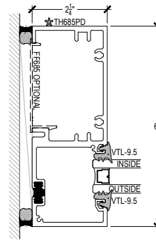
JAMB
