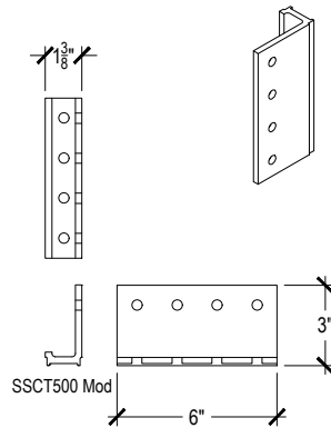
3-2 Square Bracket Jamb
