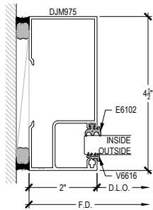
JAMB 5-1
