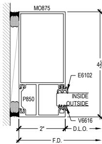
OPTIONAL JAMB 5-2
