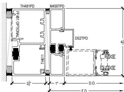
OPTIONAL THERMAL SUBFRAME DOOR JAMB
