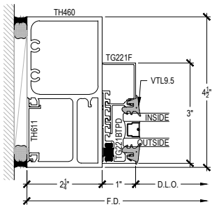
DOOR JAMB @ TRANSOM
