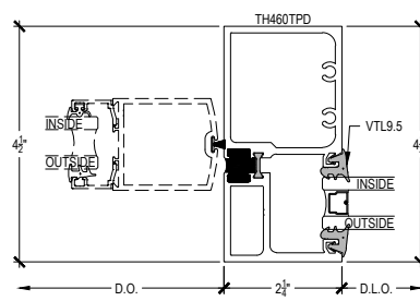
OPTIONAL THERMAL DOOR JAMB @ SIDELITE
