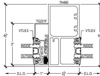
DOOR JAMB @ SIDELITE TRANSOM
