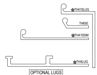
OPTIONAL LUGS
