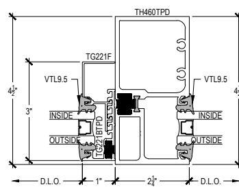
OPTIONAL THERMAL DOOR JAMB @ SIDELITE TRANSOM
